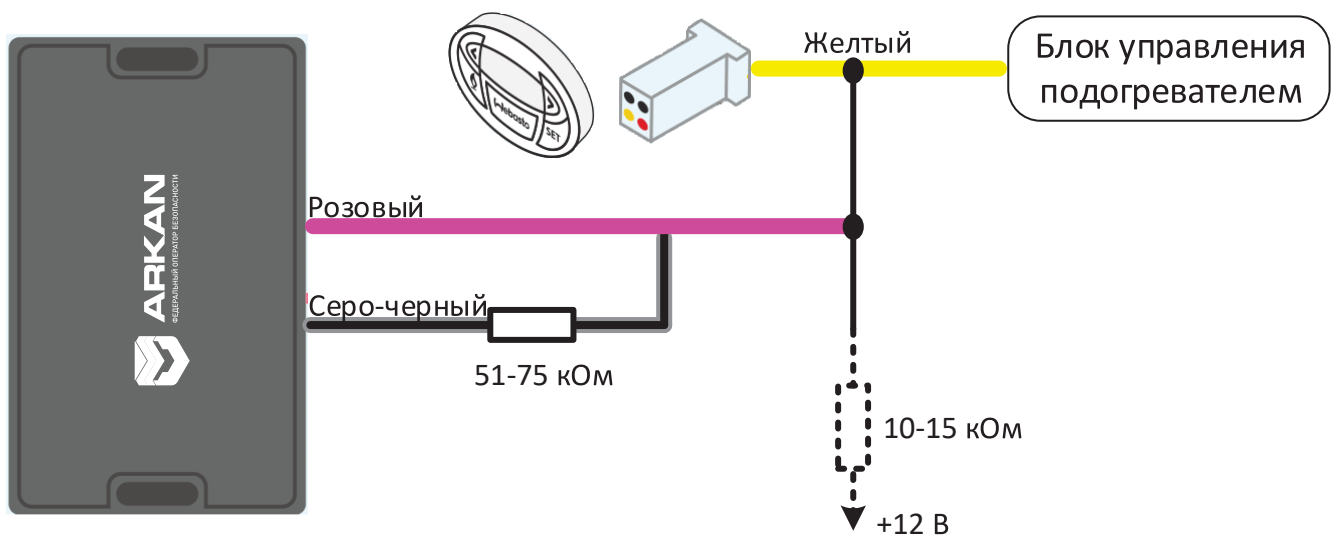
Рис.Б.2 - Схема подключения предпусковых подогревателей Webasto
